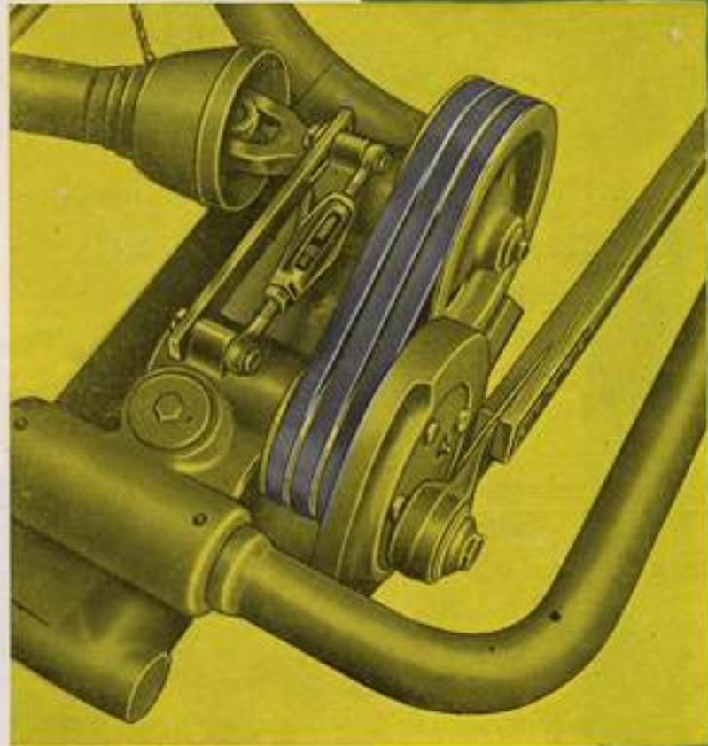
Solide Blockkonstruktion für Mähantrieb und Schleppstangenlagerung
